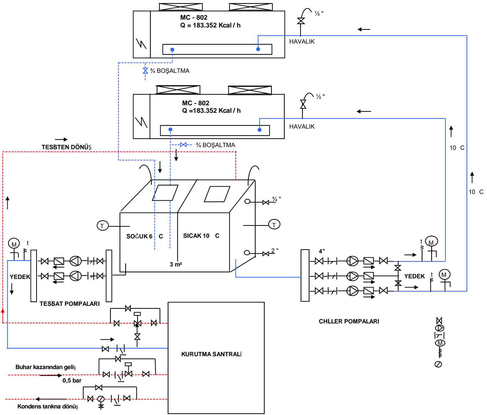
AÇIK TP, REGÜLASYON TANKLI, PROSES SANTRALLİ CHILLER, CHILLER POMPALARI, TESSAT POMPALARI, BAĞLANTI PRENSP ŞEMASI
